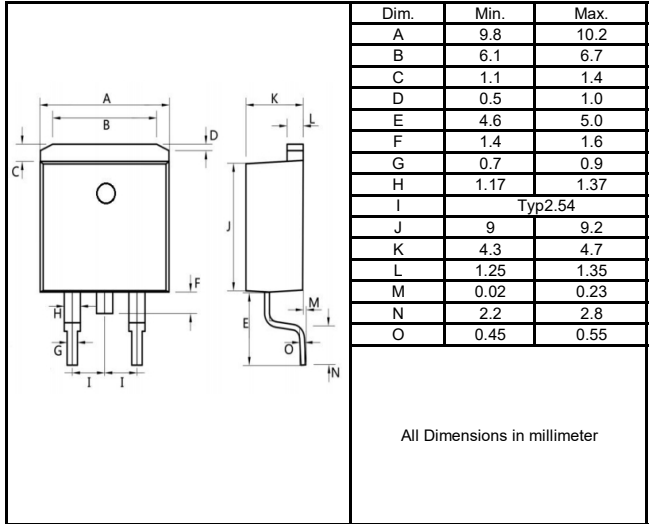
TO-263C
